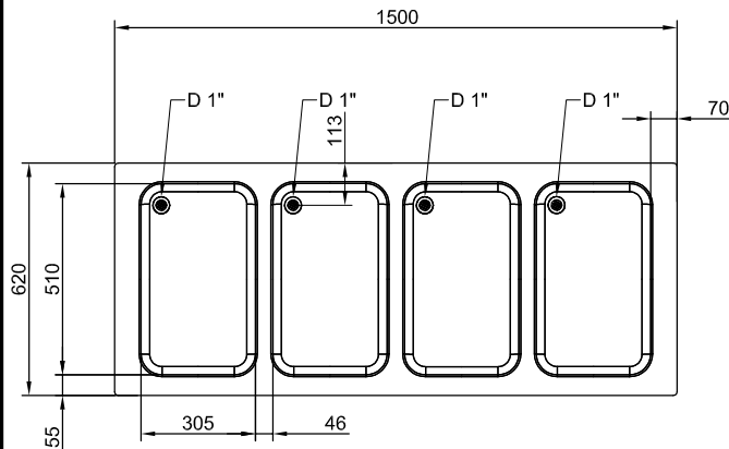
Boven aanzicht
