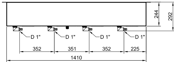
Zij aanzicht
